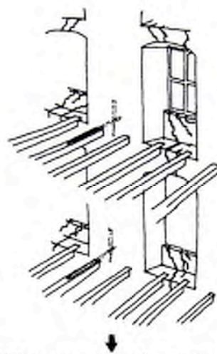
Sprickbildningens system: fönsterbröstningarna och den skevande karmen tar som svagaste element mellan murpelarna upp spänningarna i grunden. Sprickorna uppträder helt naturligt i detta område.
